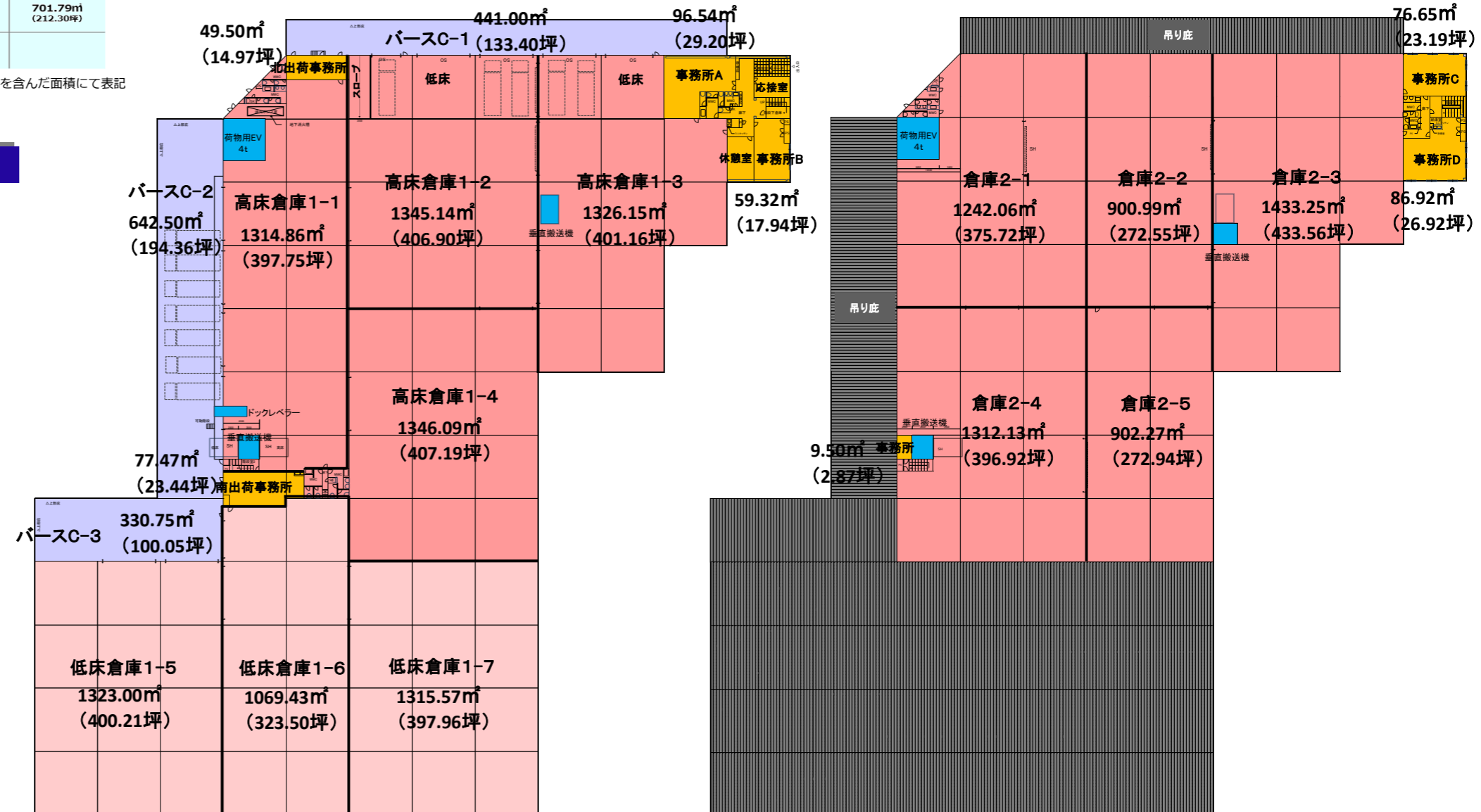
1階平面図
