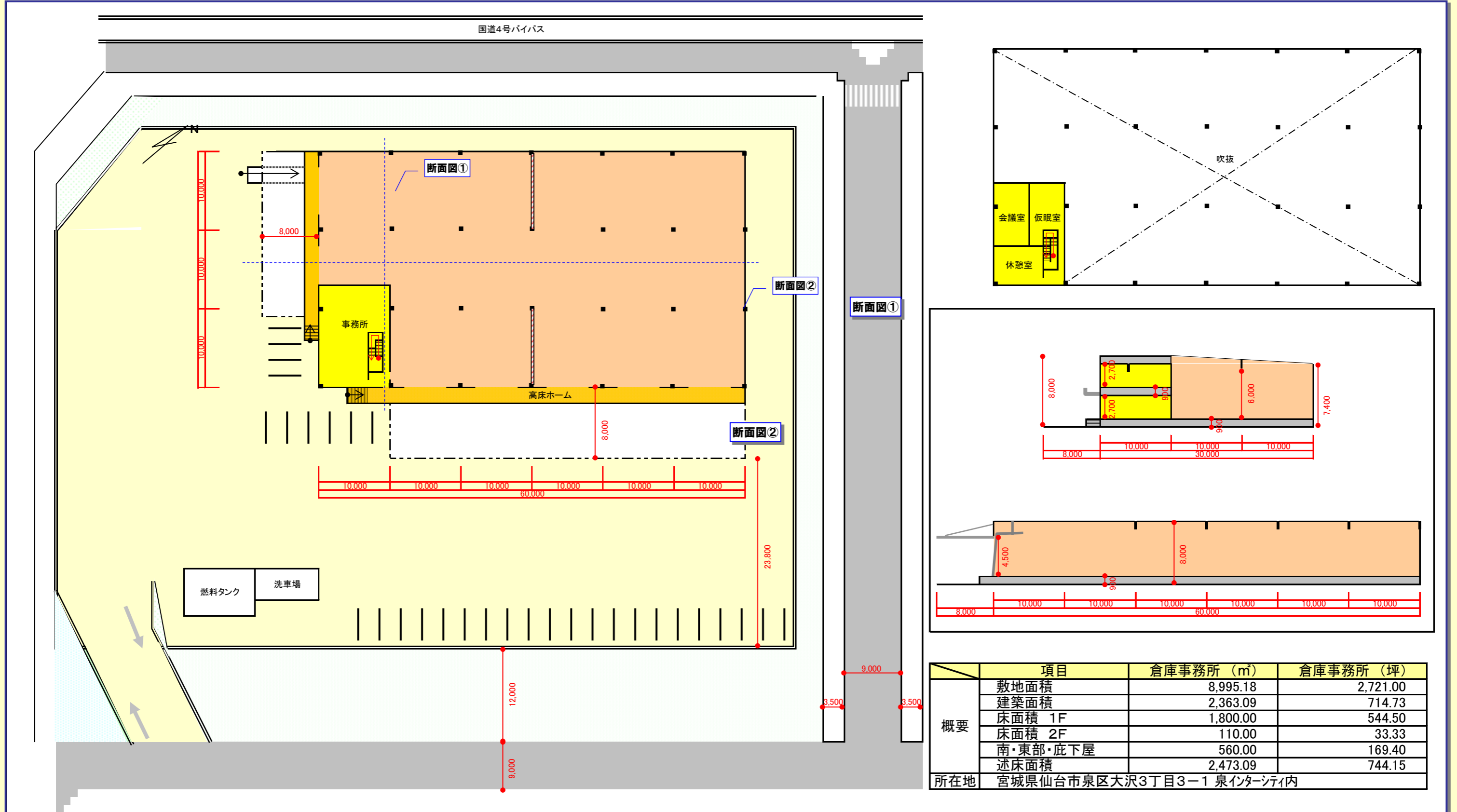
1階平面図
