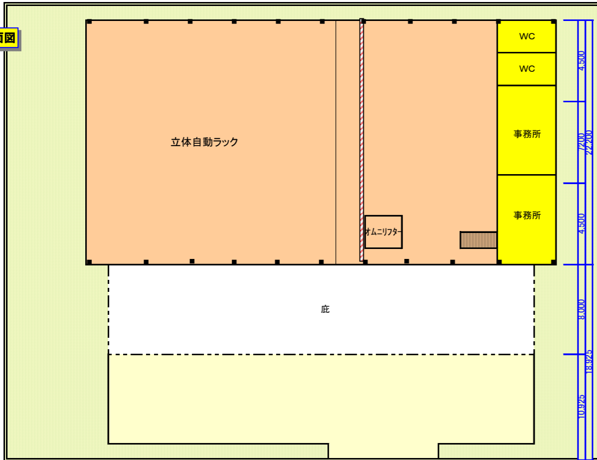
2階平面図
