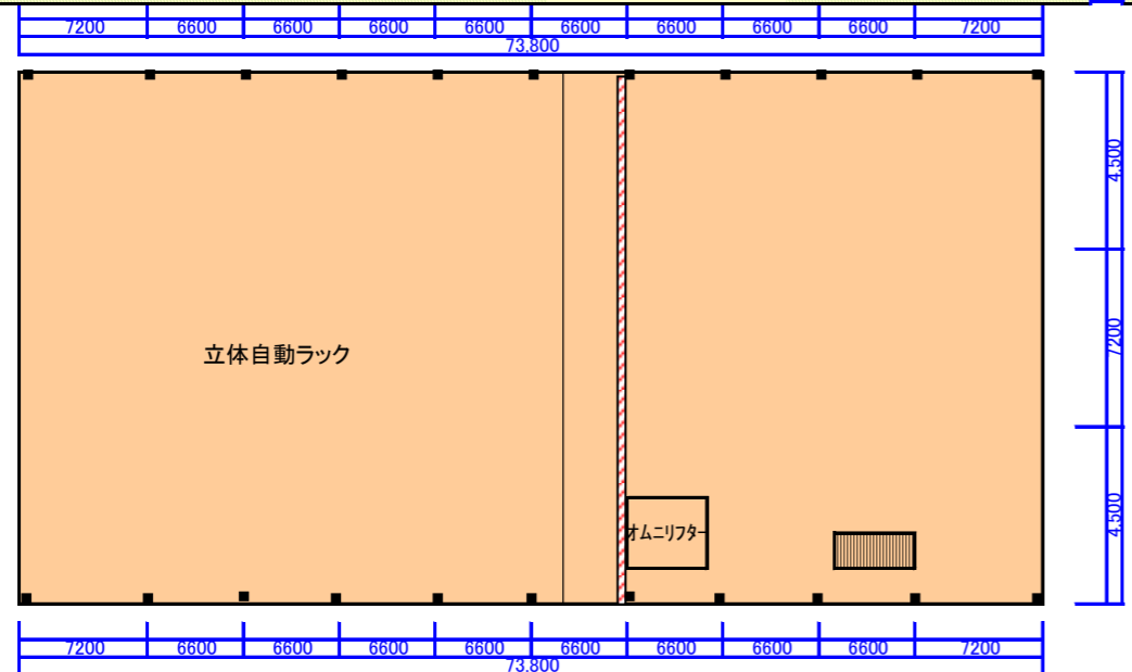
2階平面図
