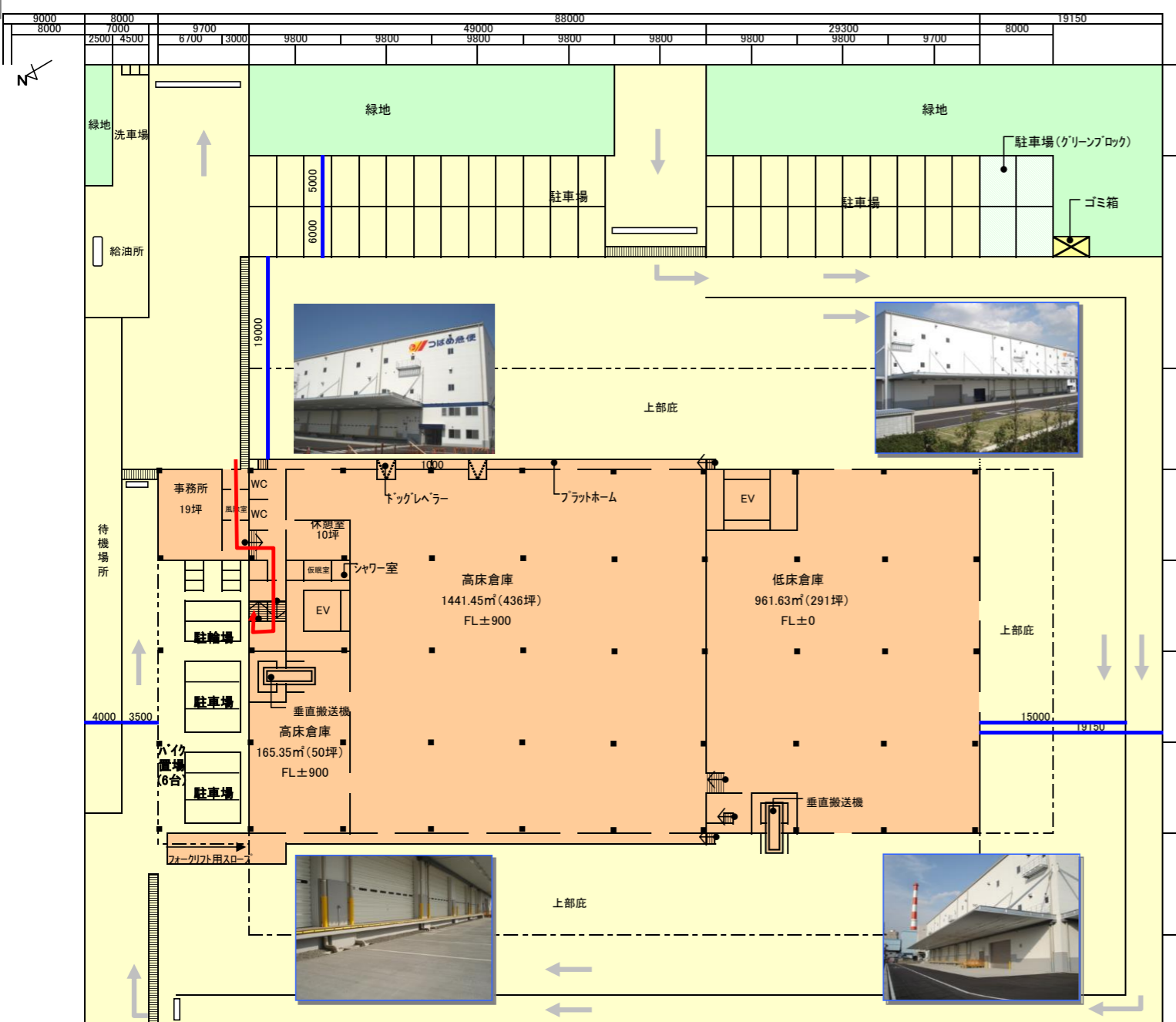
1階平面図
